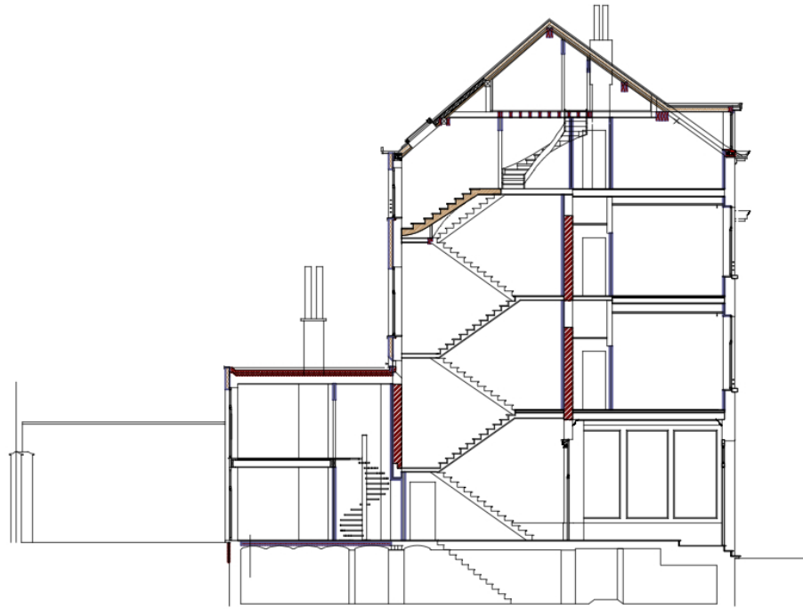
COUPE TRANSVERSALE
