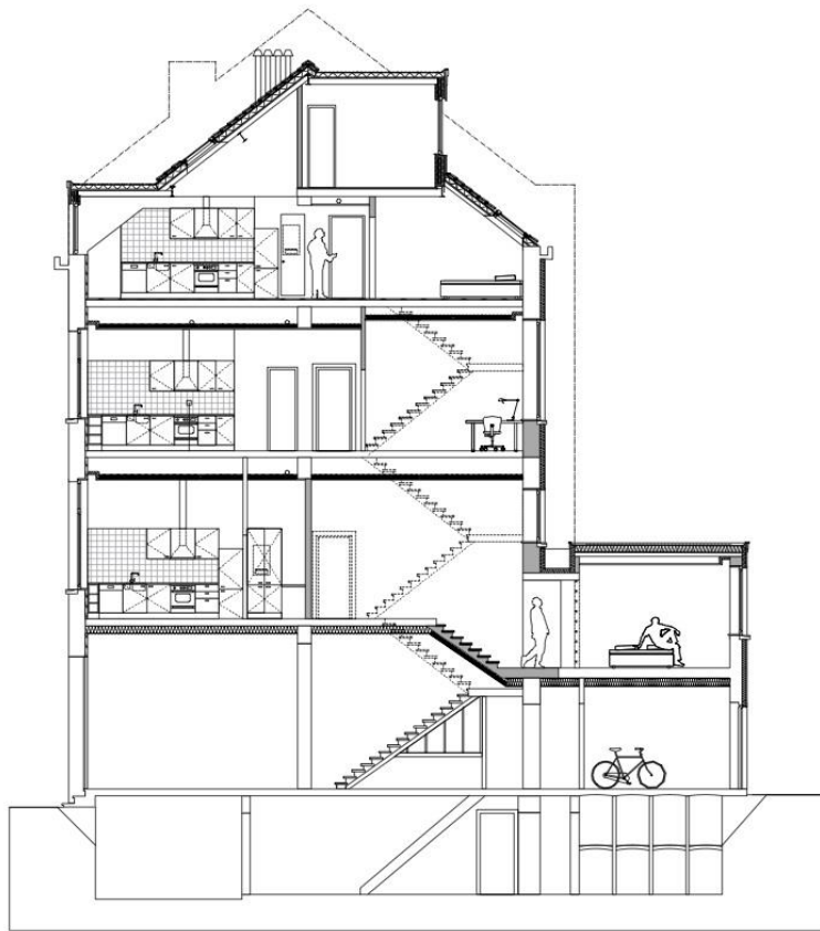
COUPE TRANSVERSALE
