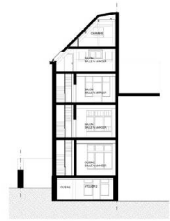
COUPE CC
