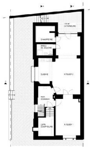
PLAN SOUS-SOL
