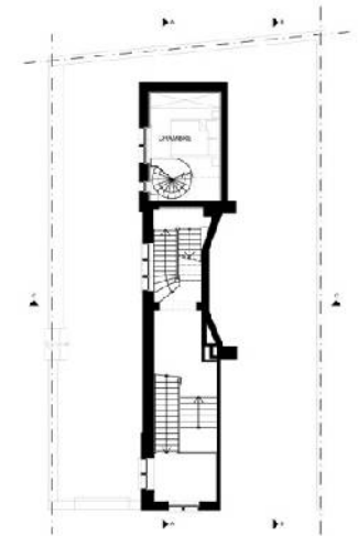
PLAN ENTRE-SOL
